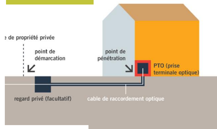
En souterrain
